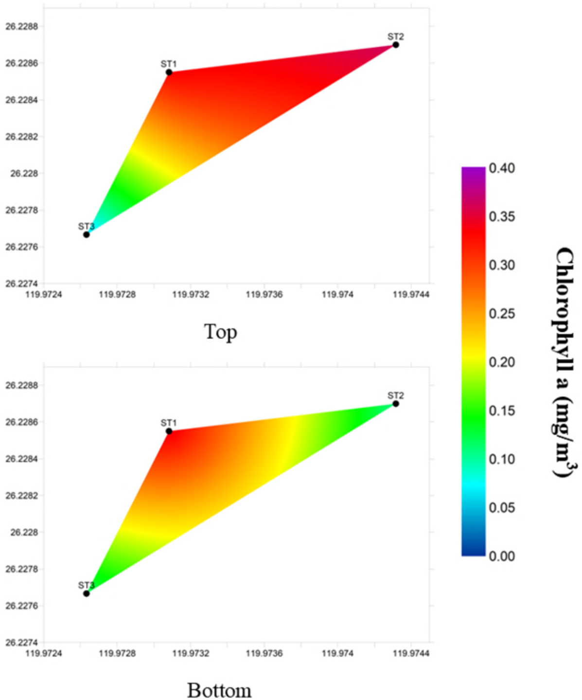
圖 23 第一次海域調查沈船處葉綠素 a 分布圖(Top:5 m; Bottom:15 m)
