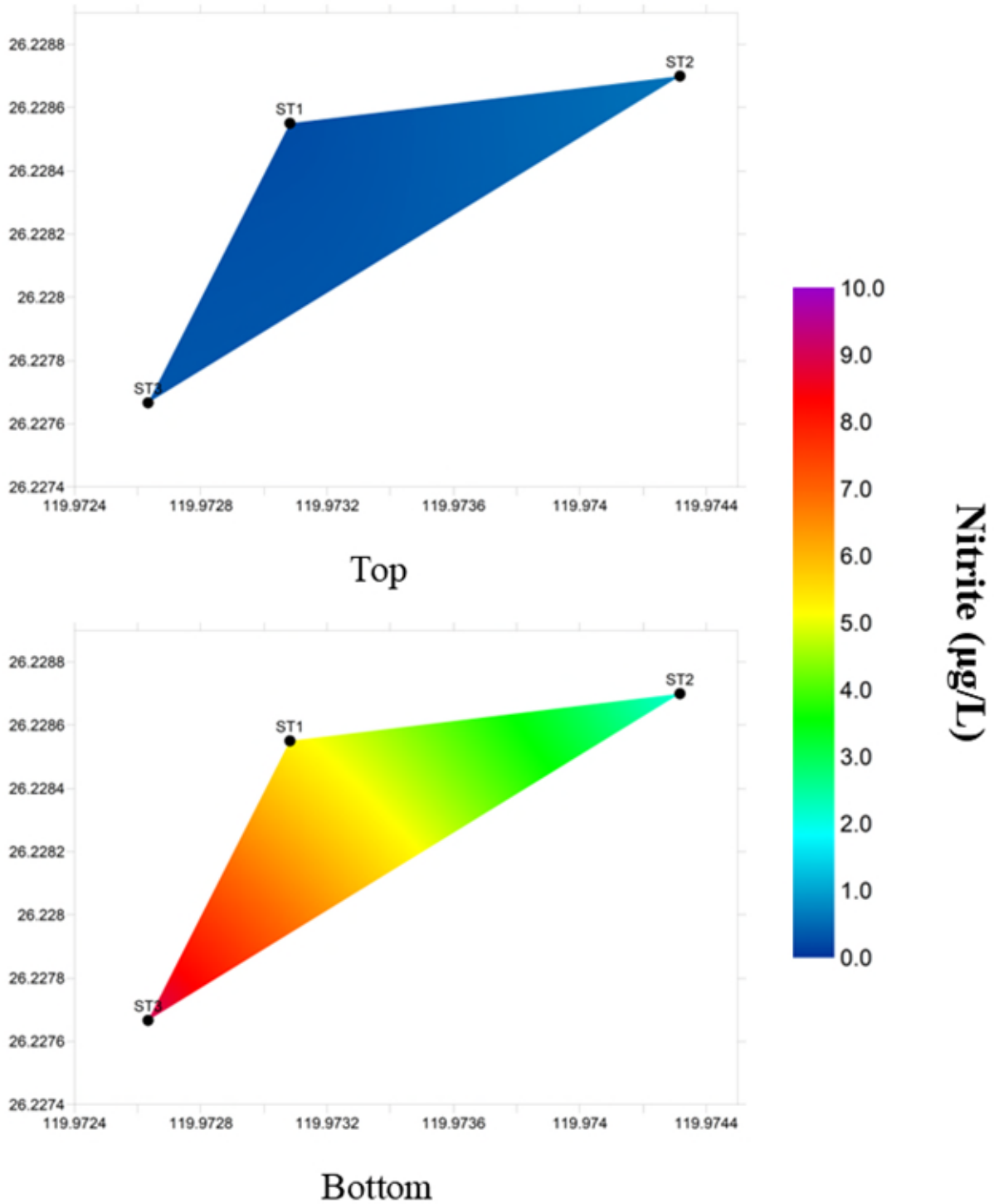
圖 20 第一次海域調查沈船處亞硝酸鹽分布圖(Top:5 m; Bottom:15 m)
