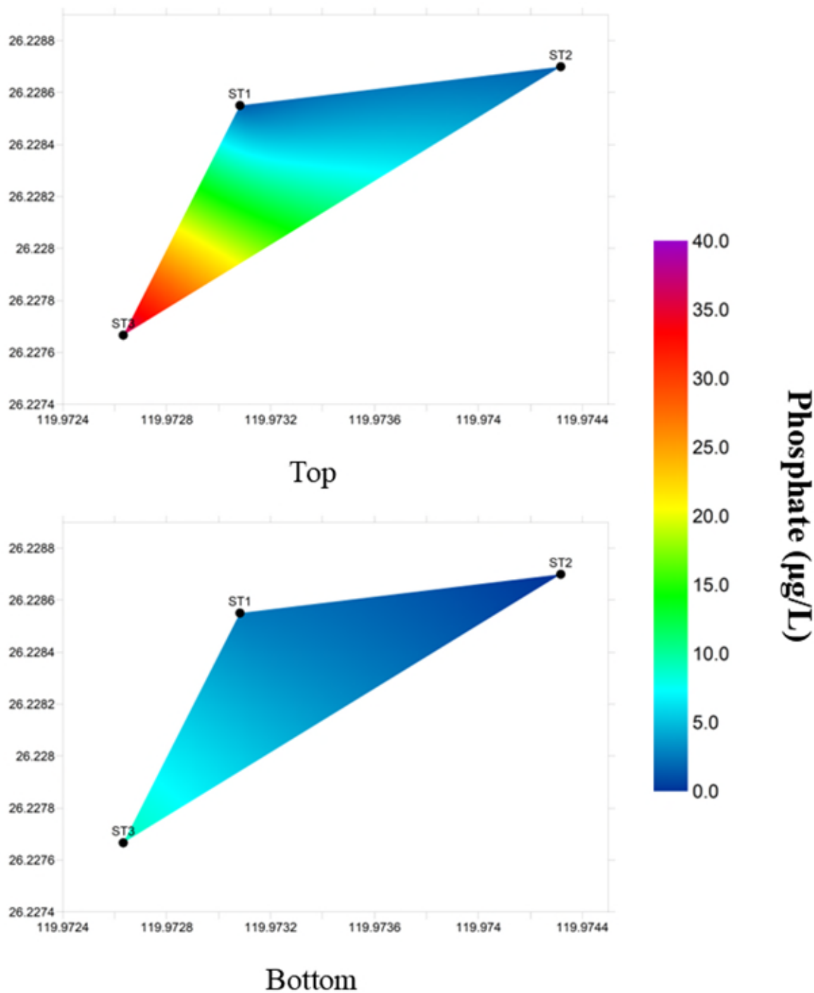
圖 21 第一次海域調查沈船處磷酸鹽分布圖(Top:5 m; Bottom:15 m)
