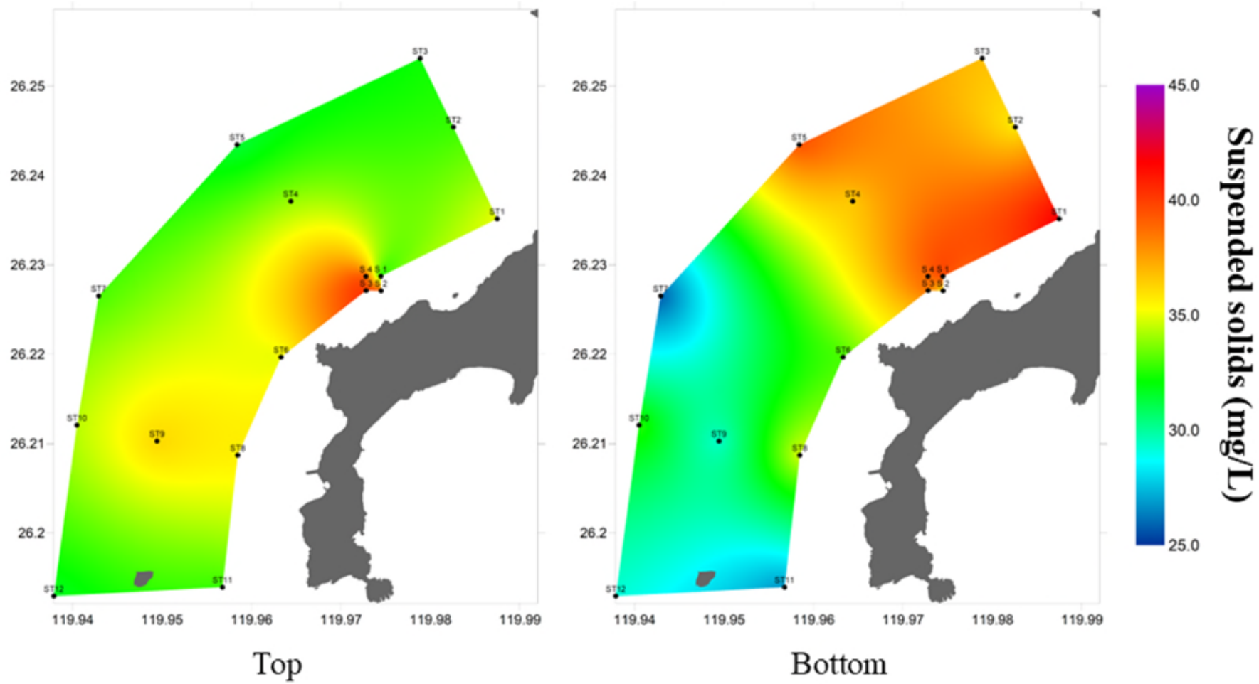
圖 28 第二次海域調查懸浮固體分布圖(Top:5 m; Bottom:15-25 m)
