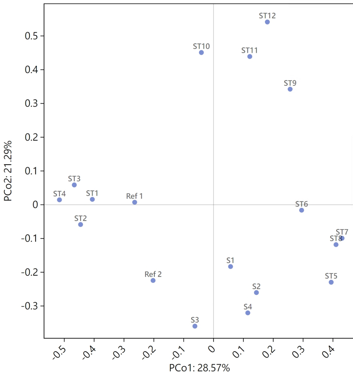
圖 12 利用主座標分析(PCoA)分析比較各測站 18 個不同測間的物種組成的相似性
