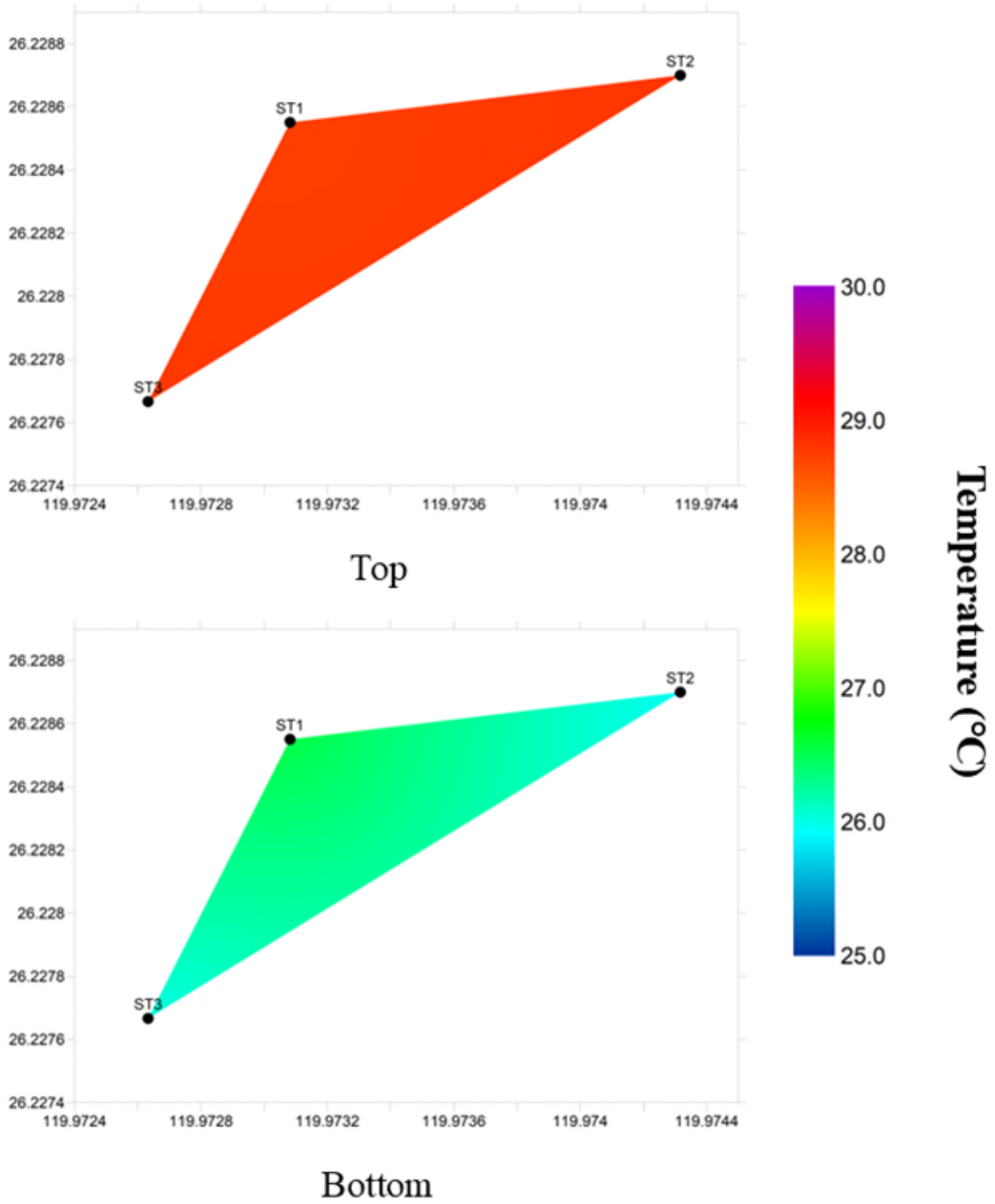
圖 13 第一次海域調查沈船處水溫分布圖(Top:5 m; Bottom:15 m)
