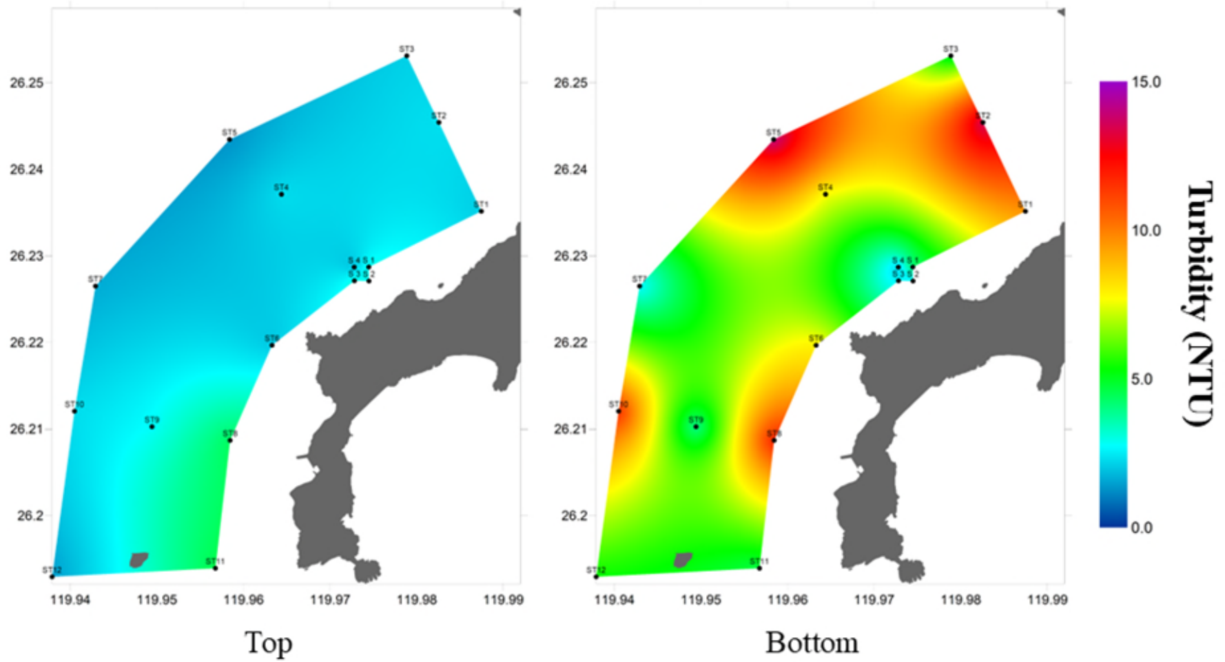
圖 29 第二次海域調查濁度分布圖(Top:5 m; Bottom:15-25 m)
