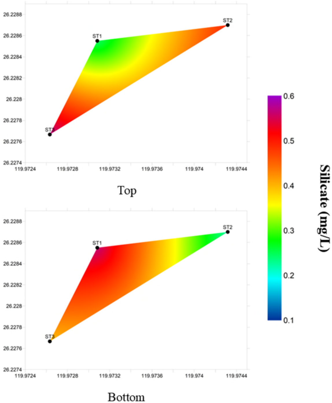
圖 22 第一次海域調查沈船處矽酸鹽分布圖(Top:5 m; Bottom:15 m)
