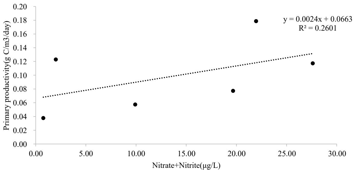
圖 41 南測線基礎生產力(g C/m 3 /day)與硝酸鹽及亞硝酸鹽總和(µg/L)之關係圖
