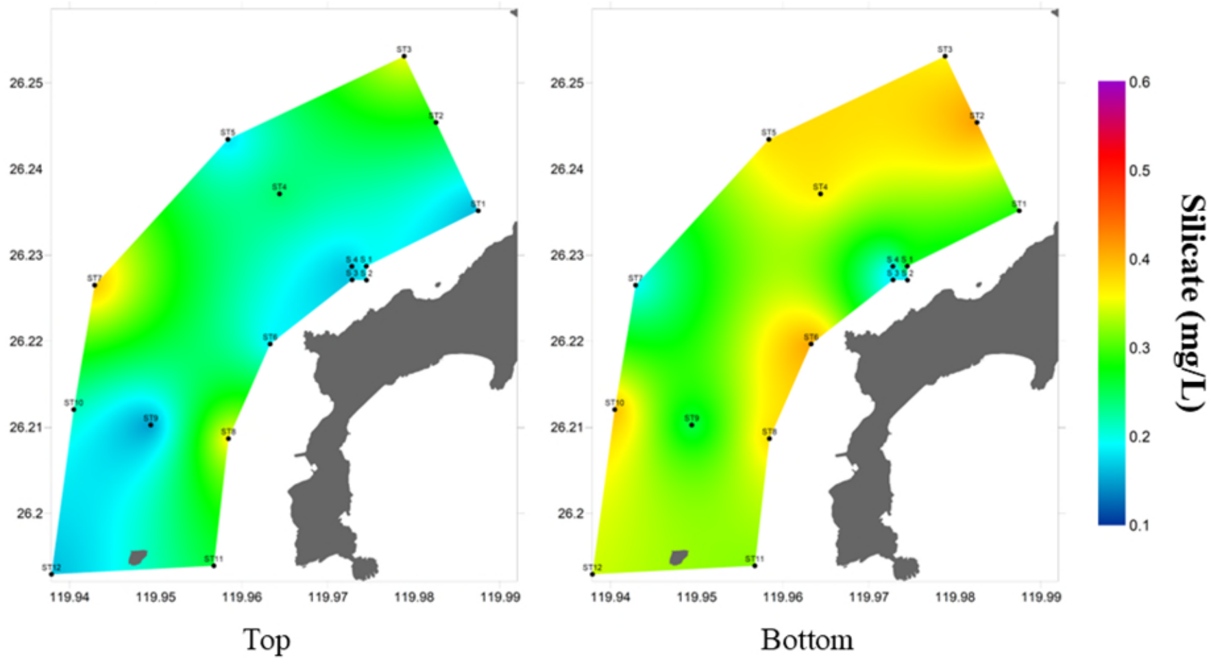
圖 34 第二次海域調查矽酸鹽分布圖(Top:5 m; Bottom:15-25 m)
