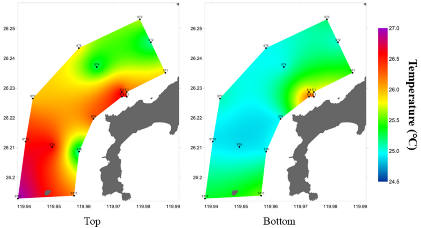
圖 25 第二次海域調查溫度分布圖(Top:5 m; Bottom:15-25 m)
