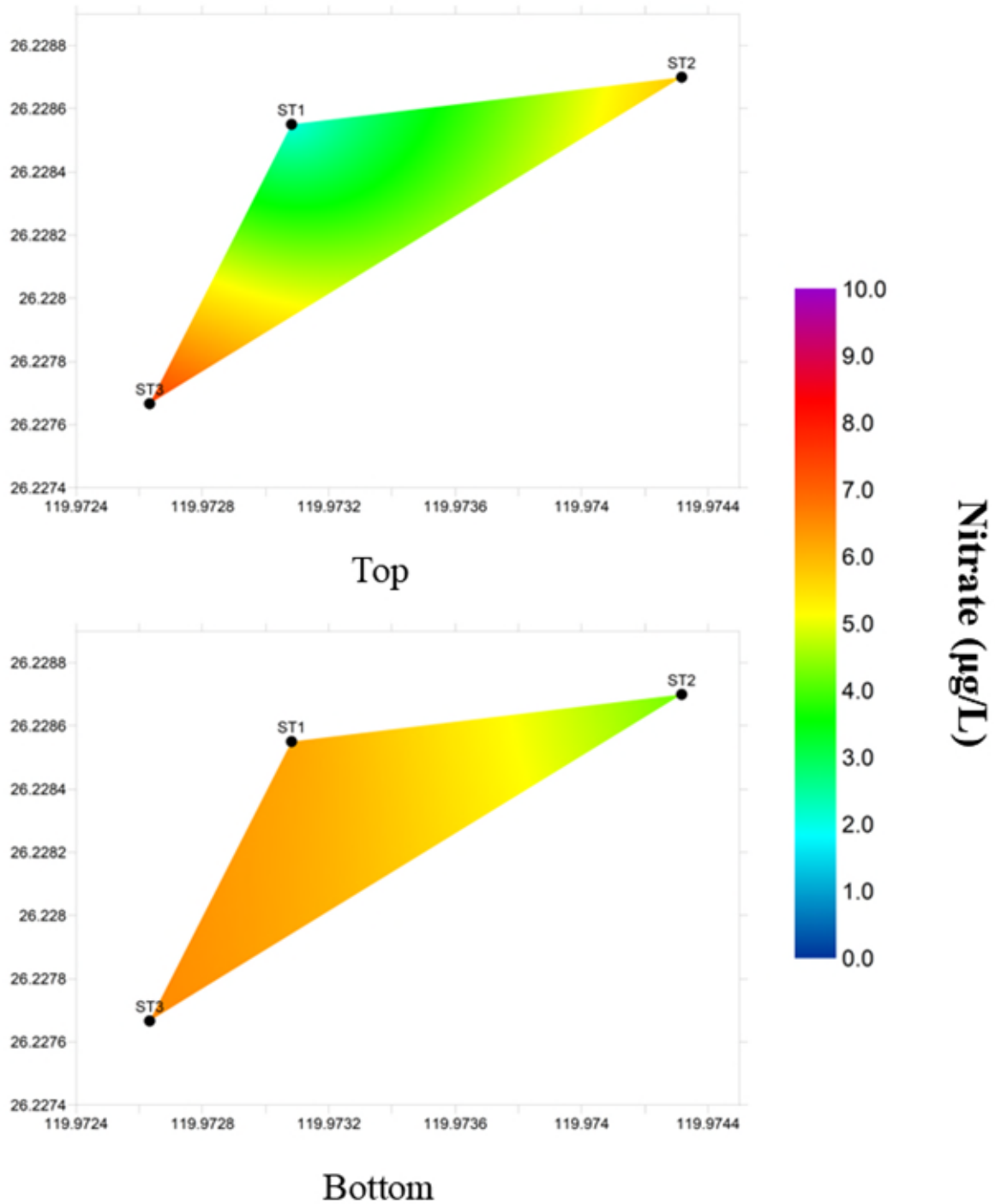
圖 19 第一次海域調查沈船處硝酸鹽分布圖(Top:5 m; Bottom:15 m)
