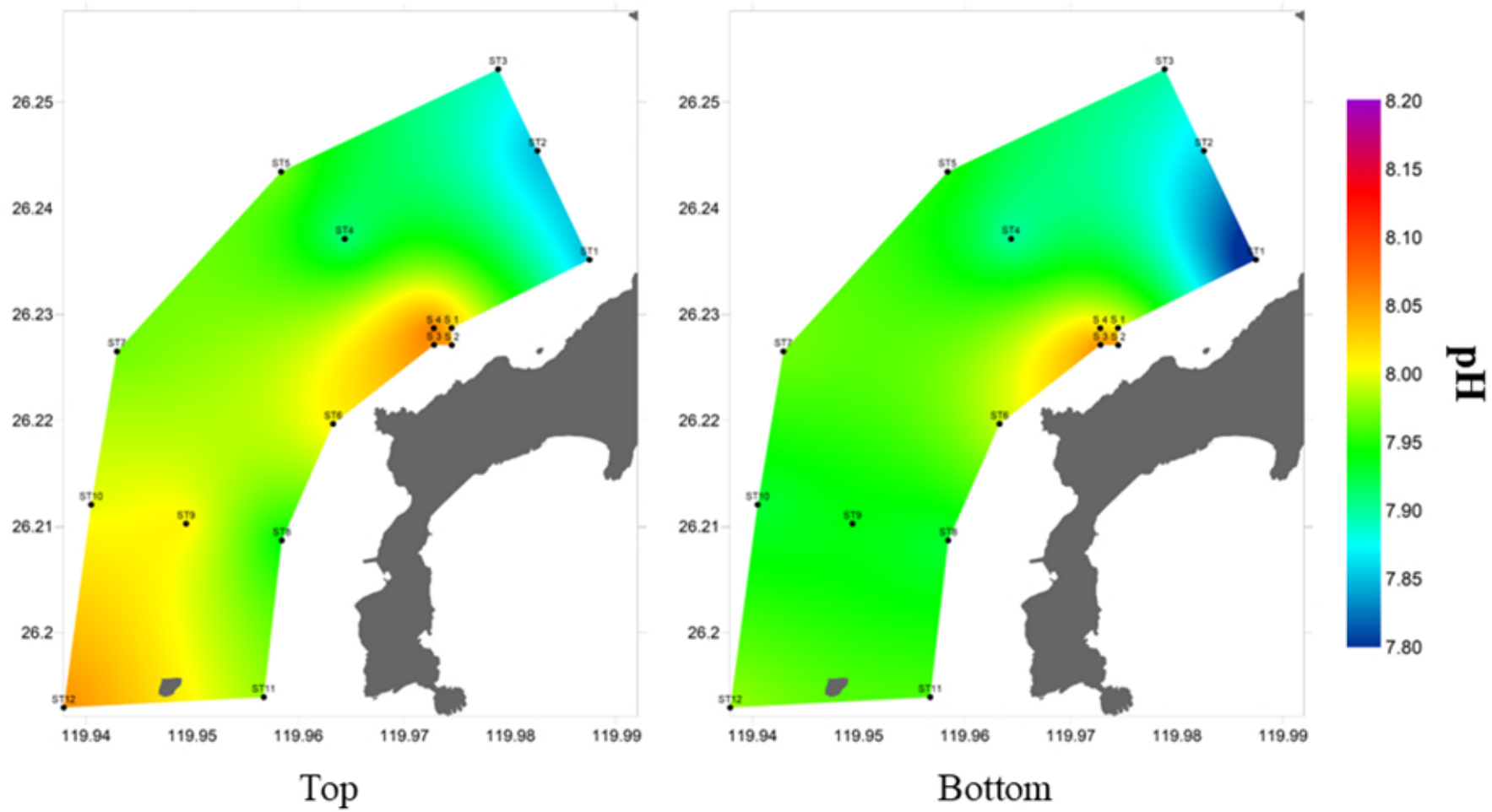
圖 27 第二次海域調查 pH 分布圖(Top:5 m; Bottom:15-25 m)
