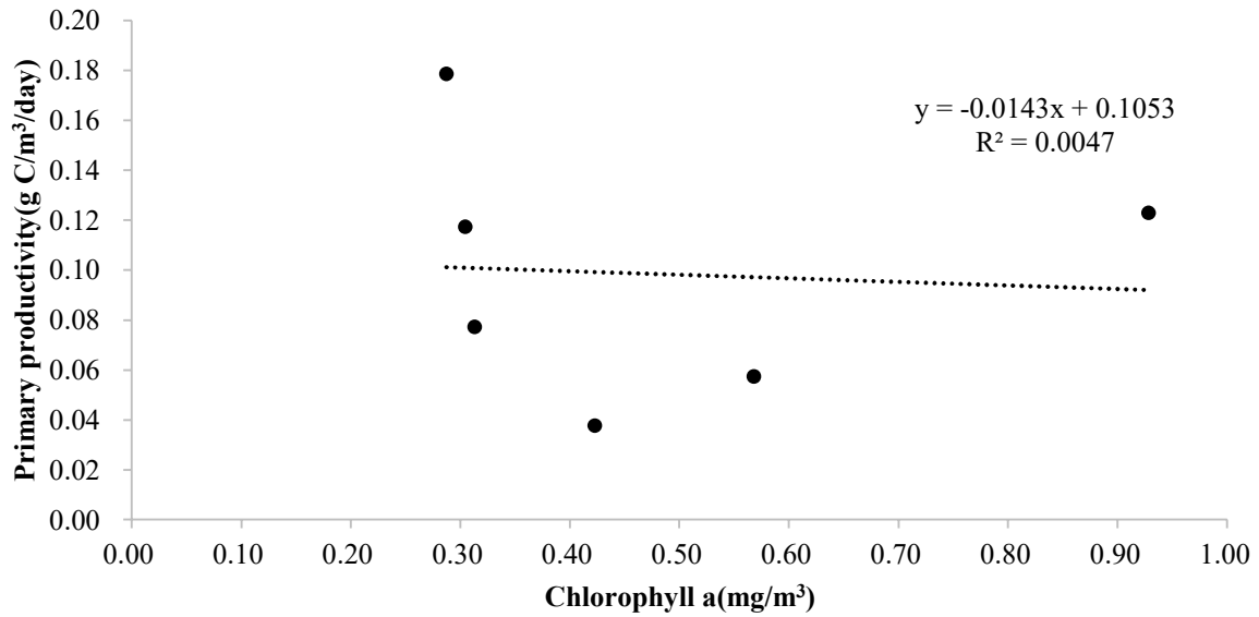
圖 46 南測線葉綠素 a(mg/m 3 )與基礎生產力(g C/m 3 /day)之關係圖
