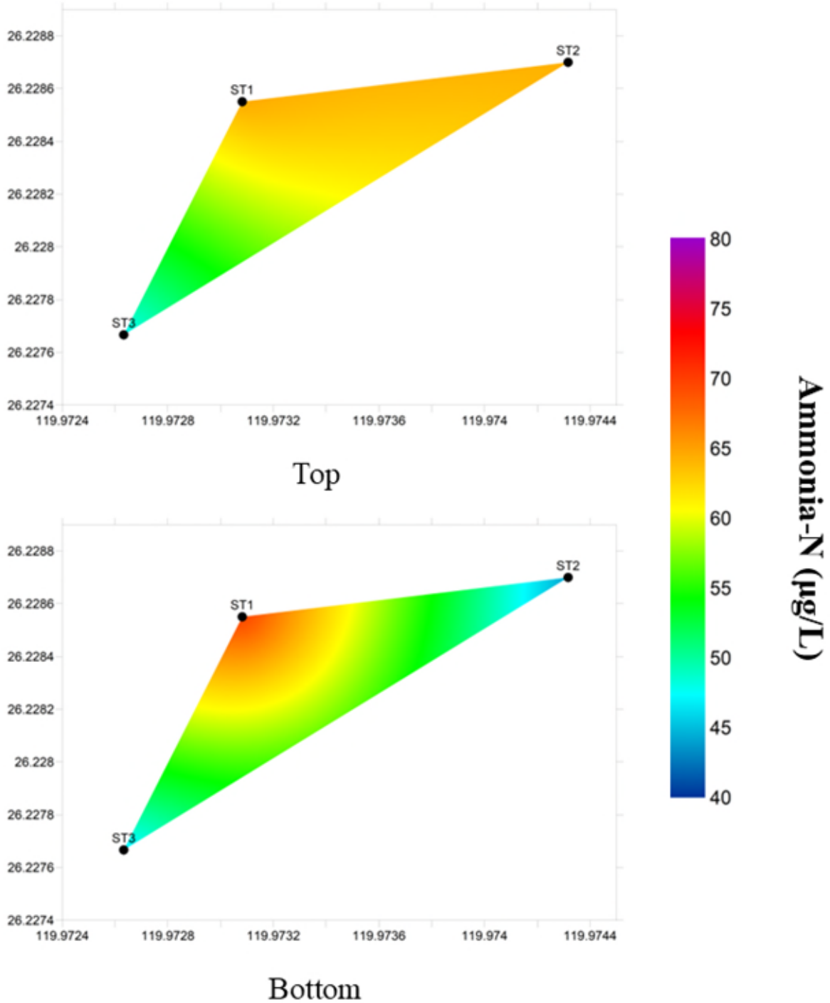
圖 18 第一次海域調查沈船處氨-氮分布圖(Top:5 m; Bottom:15 m)
