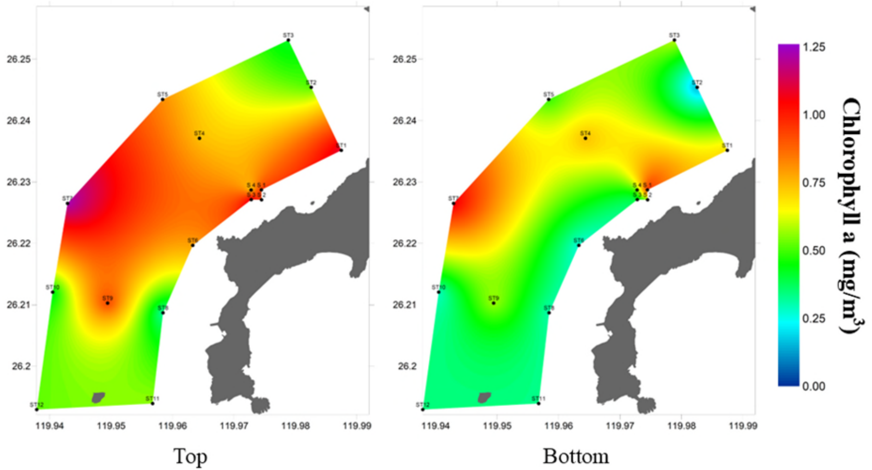
圖 35 第二次海域調查葉綠素 a 分布圖(Top:5 m; Bottom:15-25 m)
