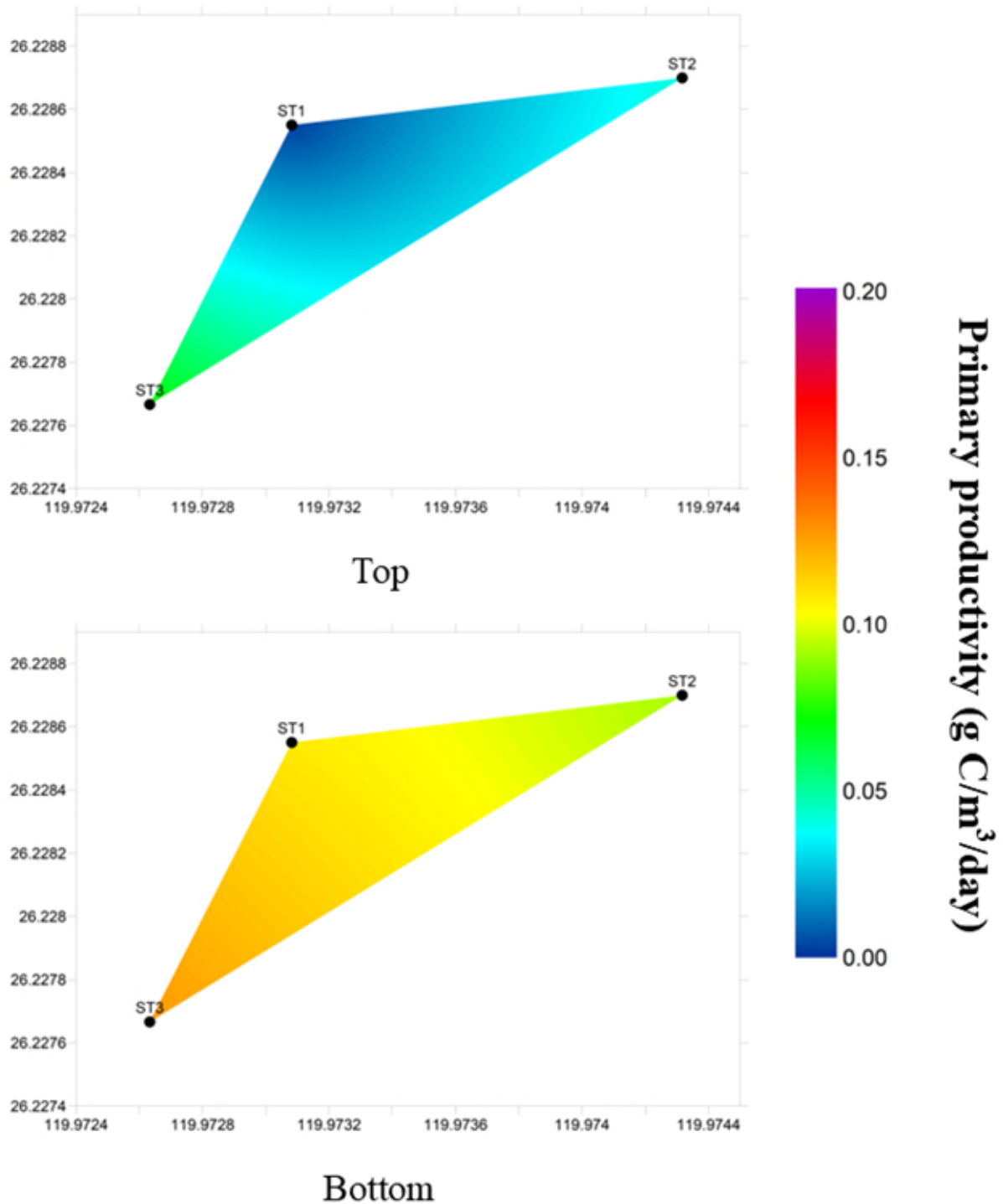
圖 24 第一次海域調查沈船處基礎生產力分布圖(Top:5 m; Bottom:15 m)
