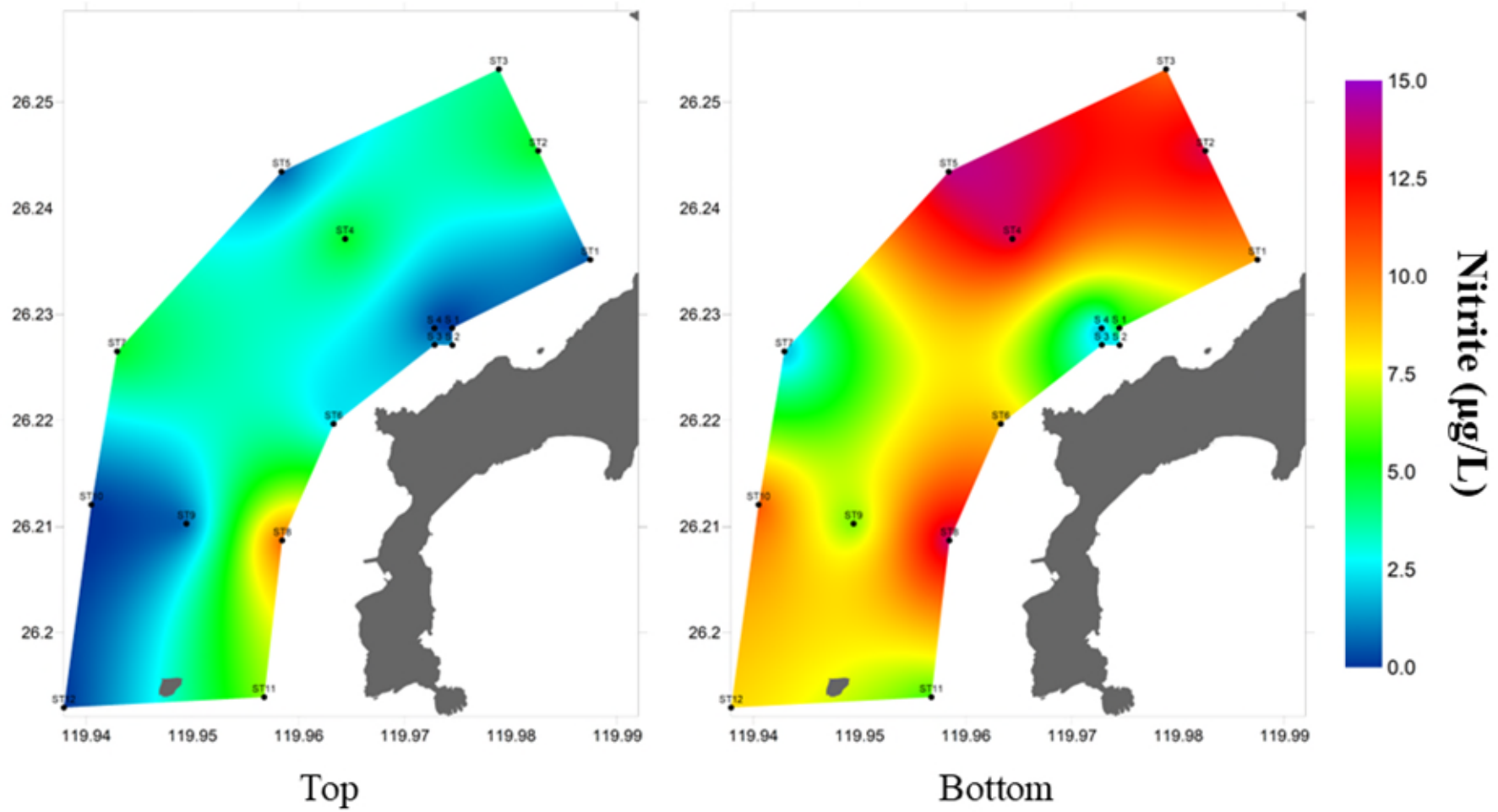
圖 32 第二次海域調查亞硝酸鹽分布圖(Top:5 m; Bottom:15-25 m)
