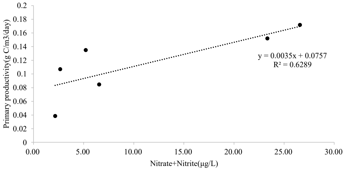
圖 40 中測線基礎生產力(g C/m 3 /day)與硝酸鹽及亞硝酸鹽總和(µg/L)之關係圖
