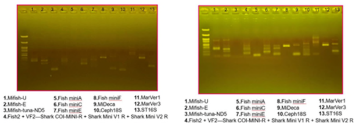
圖 10 初步利用臺灣東北角開放海域收集水體 eDNA 檢體 PCR 反應
