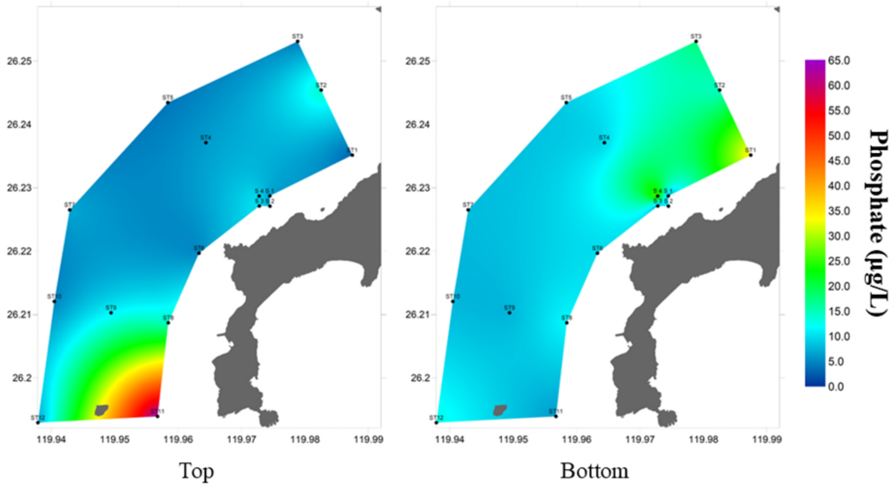
圖 33 第二次海域調查磷酸鹽分布圖(Top:5 m; Bottom:15-25 m)
