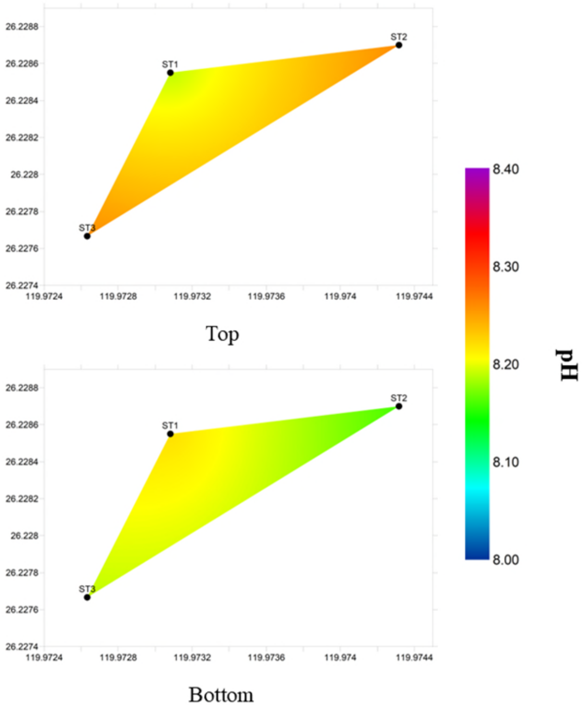
圖 15 第一次海域調查沈船處 pH 值分布圖(Top:5 m; Bottom:15 m)
