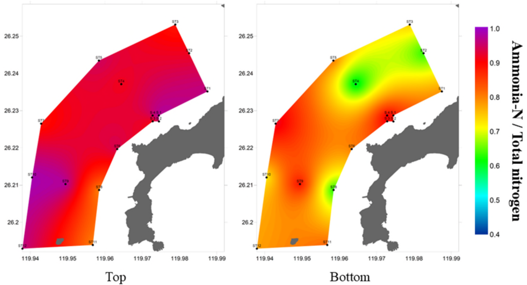
圖 37 第二次海域調查氨-氮/總氮分布圖(Top:5 m; Bottom:15-25 m)
