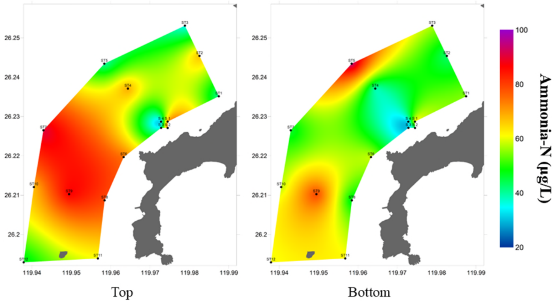
圖 30 第二次海域調查氨-氮分布圖(Top:5 m; Bottom:15-25 m)
