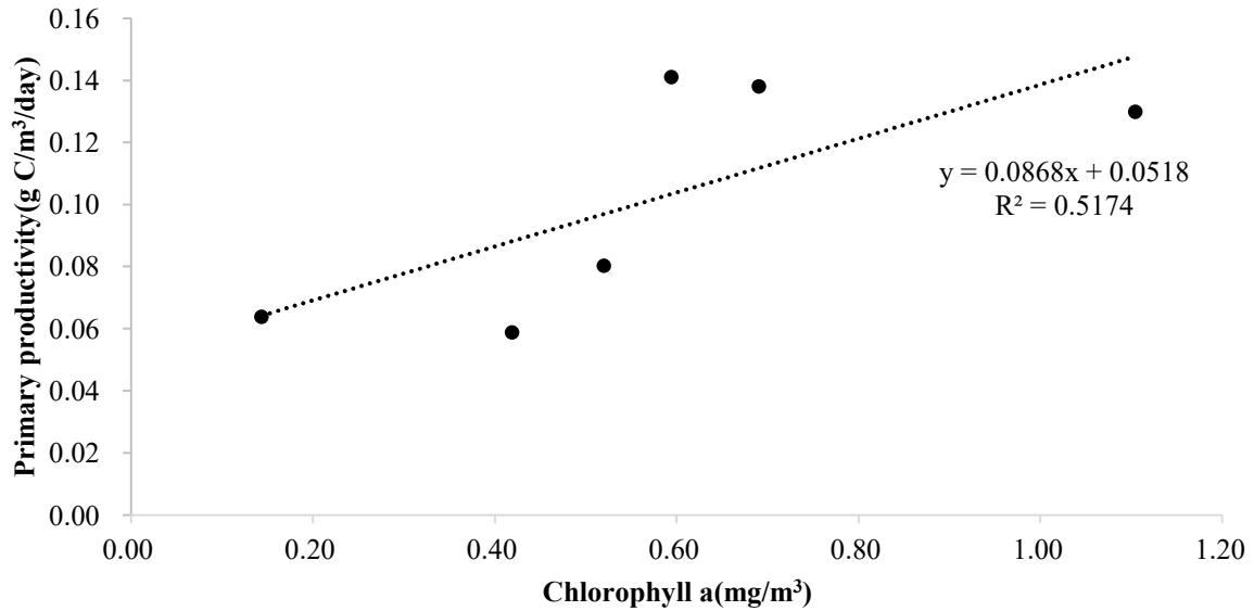
圖 44 北側線葉綠素 a(mg/m 3 )與基礎生產力(g C/m 3 /day)之關係圖
