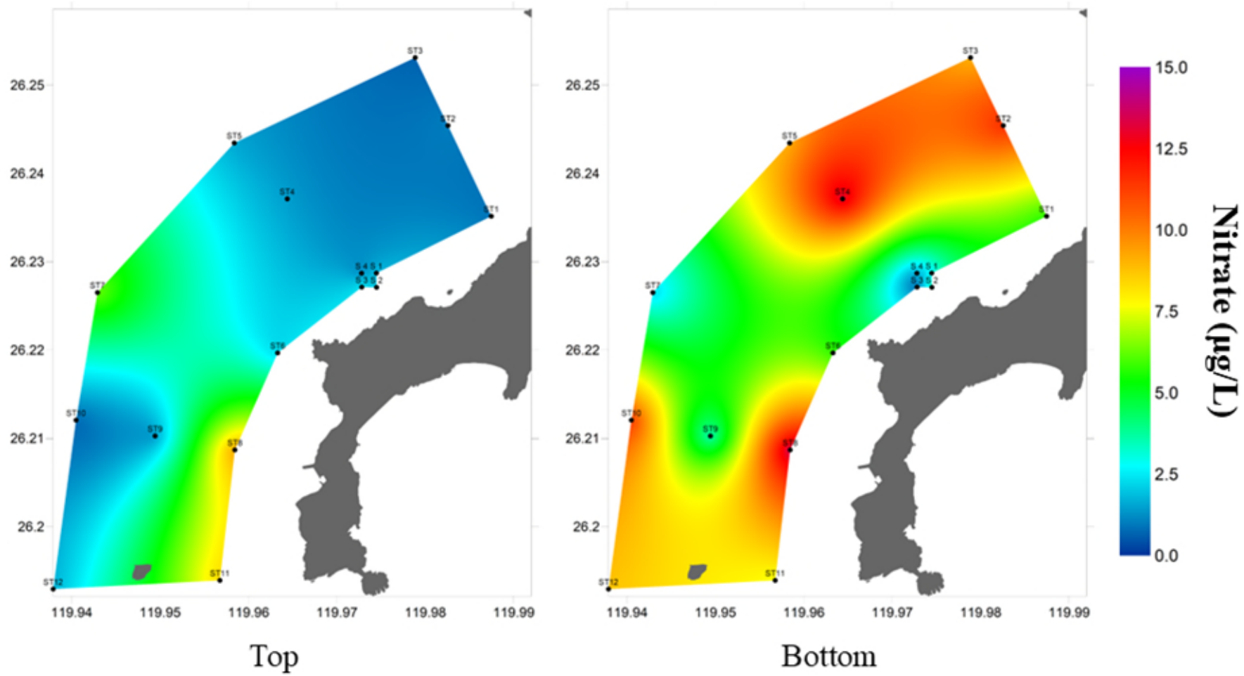
圖 31 第二次海域調查硝酸鹽分布圖(Top:5 m; Bottom:15-25 m)
