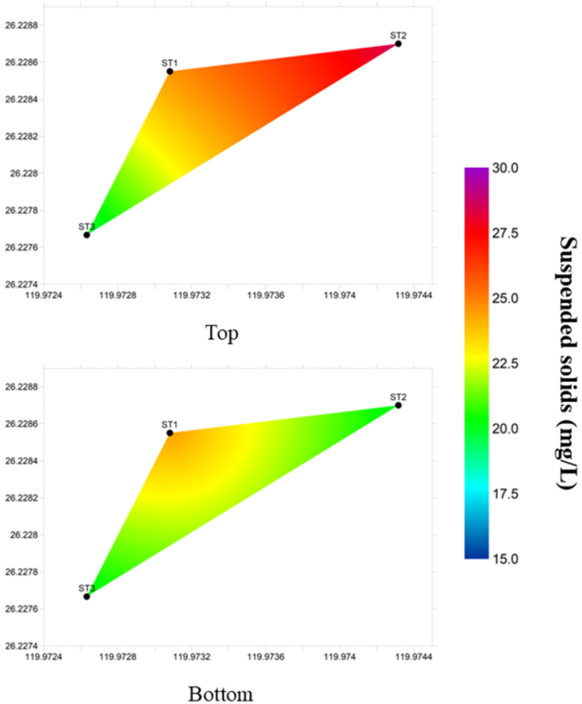
圖 16 第一次海域調查沈船處懸浮固體分布圖(Top:5 m; Bottom:15 m)
