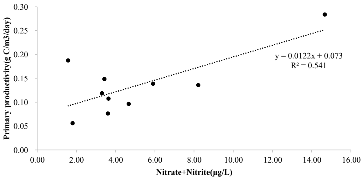
圖 43 第二次調查沈船處測站與 ST6 之基礎生產力(g C/m 3 /day)與硝酸鹽及亞硝酸鹽總和(µg/L)之關係圖
