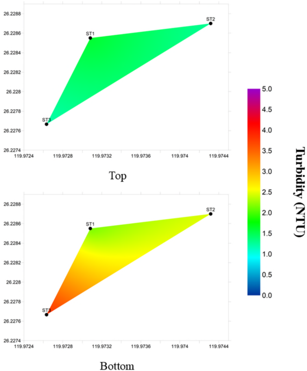
圖 17 第一次海域調查沈船處濁度分布圖(Top:5 m; Bottom:15 m)
