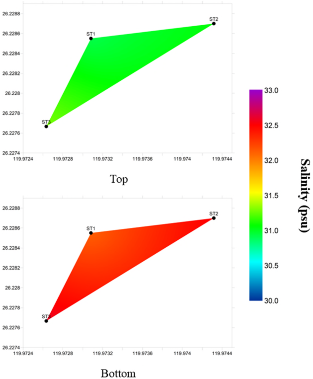
圖 14 第一次海域調查沈船處鹽度分布圖(Top:5 m; Bottom:15 m)
