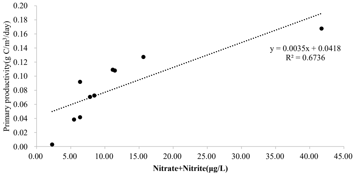
圖 42 第一次調查沈船處與參考點之基礎生產力(g C/m 3 /day)與硝酸鹽及亞硝酸鹽總和(µg/L)之關係圖
