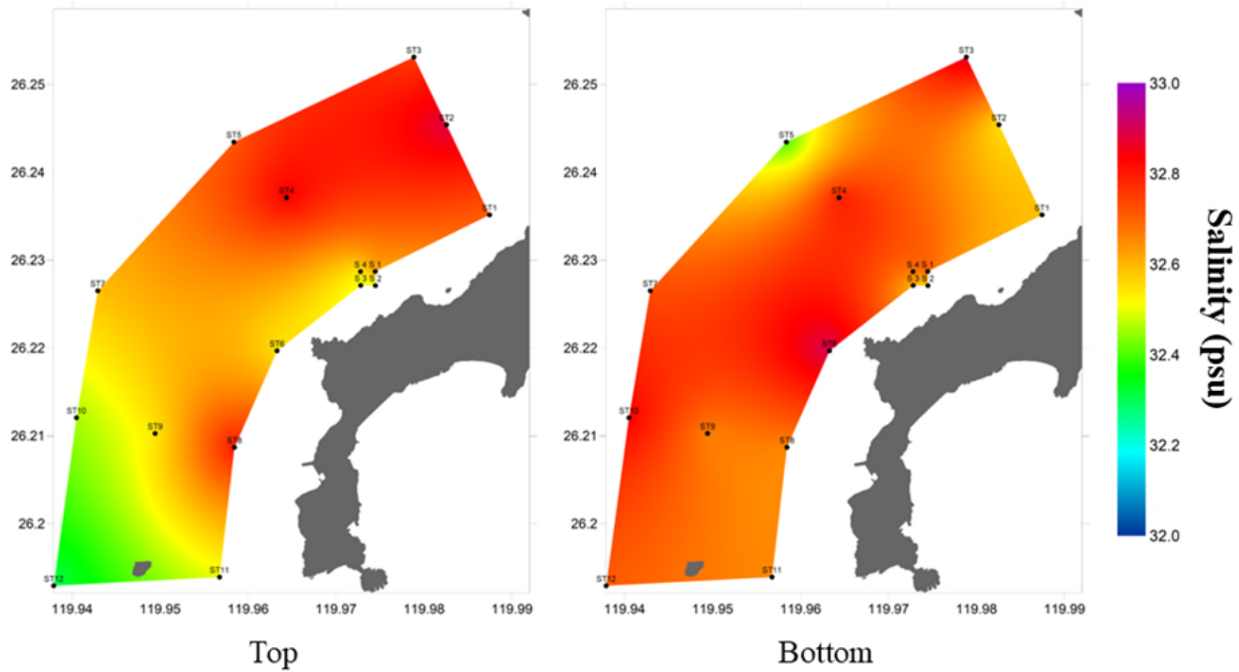
圖 26 第二次海域調查鹽度分布圖(Top:5 m; Bottom:15-25 m)
