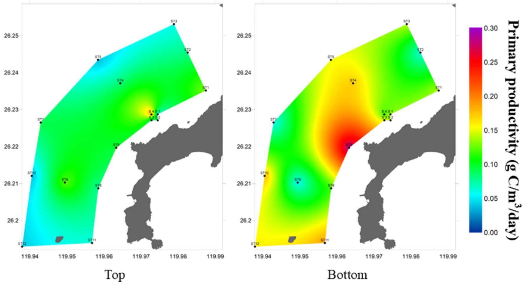
圖 36 第二次海域調查基礎生產力分布圖(Top:5 m; Bottom:15-25 m)
